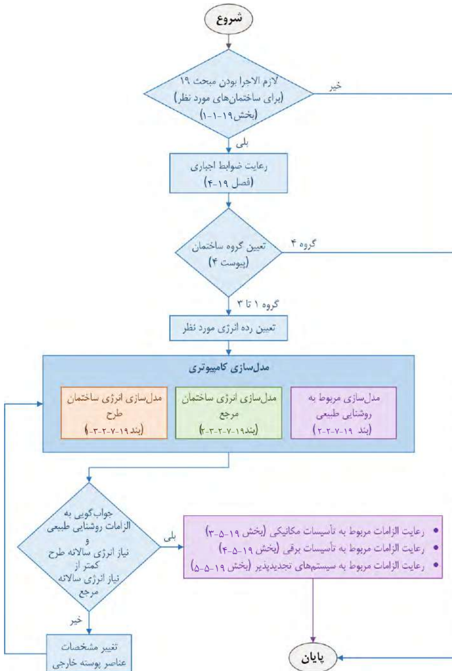
شکل ۱۹-۷-۱ نمودار گردش مراحل روش نیاز انرژی
